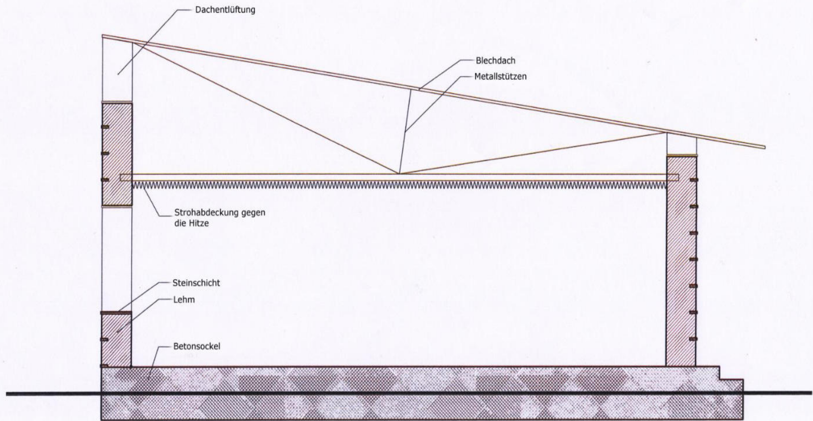
Gebäudequerschnitt
