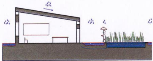
Konzept der Belüftung und der Wasserwiederaufbereitung
